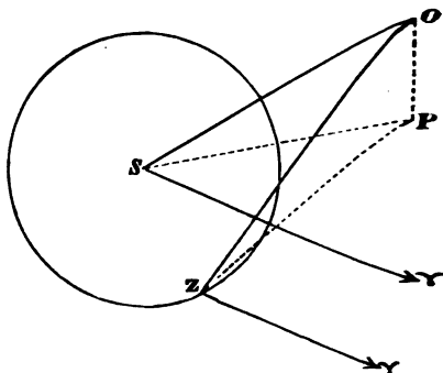
Č. 1675. Heliocentrická délka a šířka.
